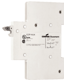
CCP-AUX
